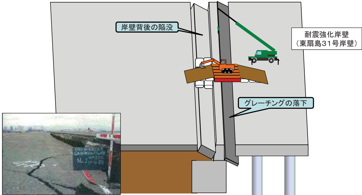
岸壁背後の陥没
